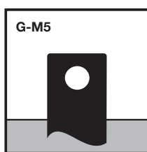
Под винт G-5 мм, 5 Nm
