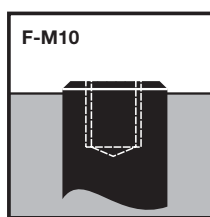
Винт F-M10, 17 Nm
